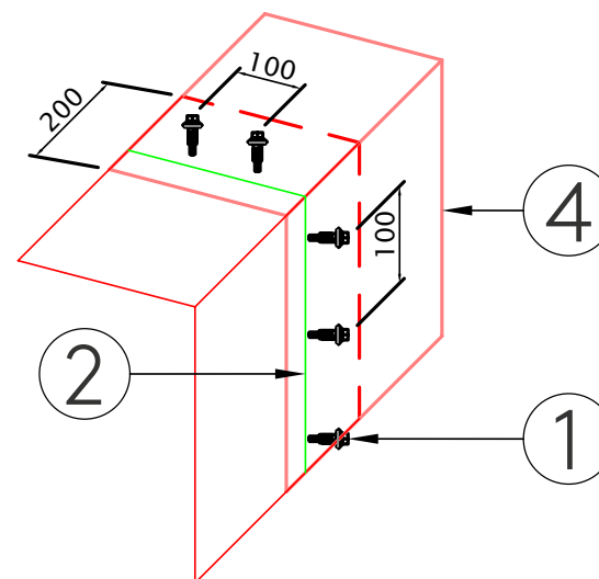
Exemplo de costura transversal de rufos
