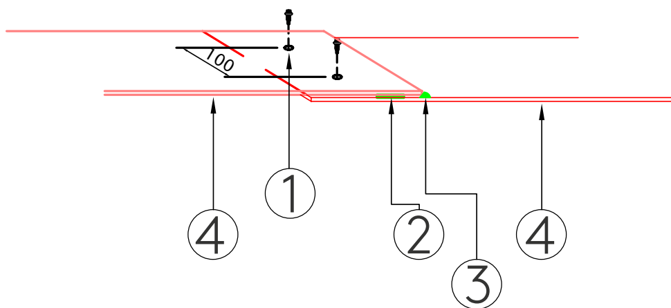
Detalhe padrão de costura transversal de rufos
