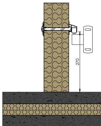
SEÇÃO A-A
